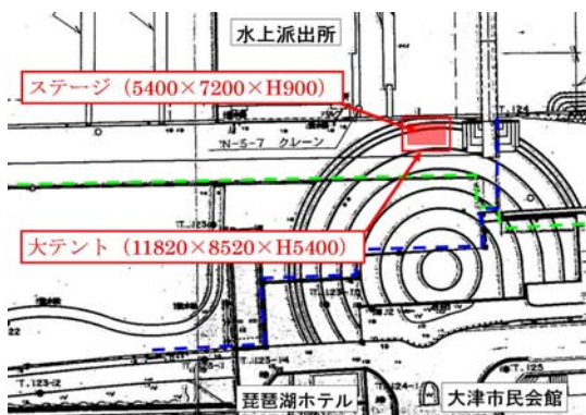
大テント（11820×8520×H5400）、ステージ（5400×7200×H900）
